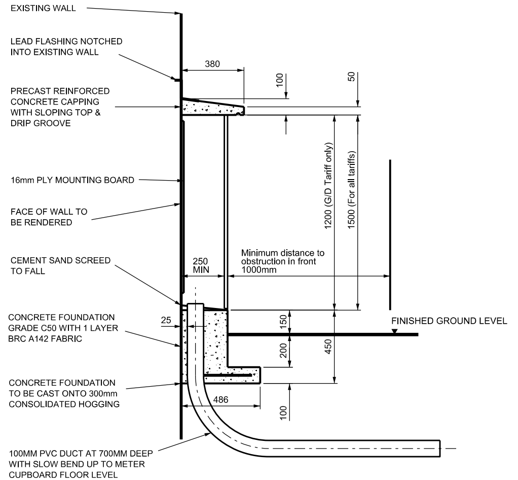
SECTION A-A
