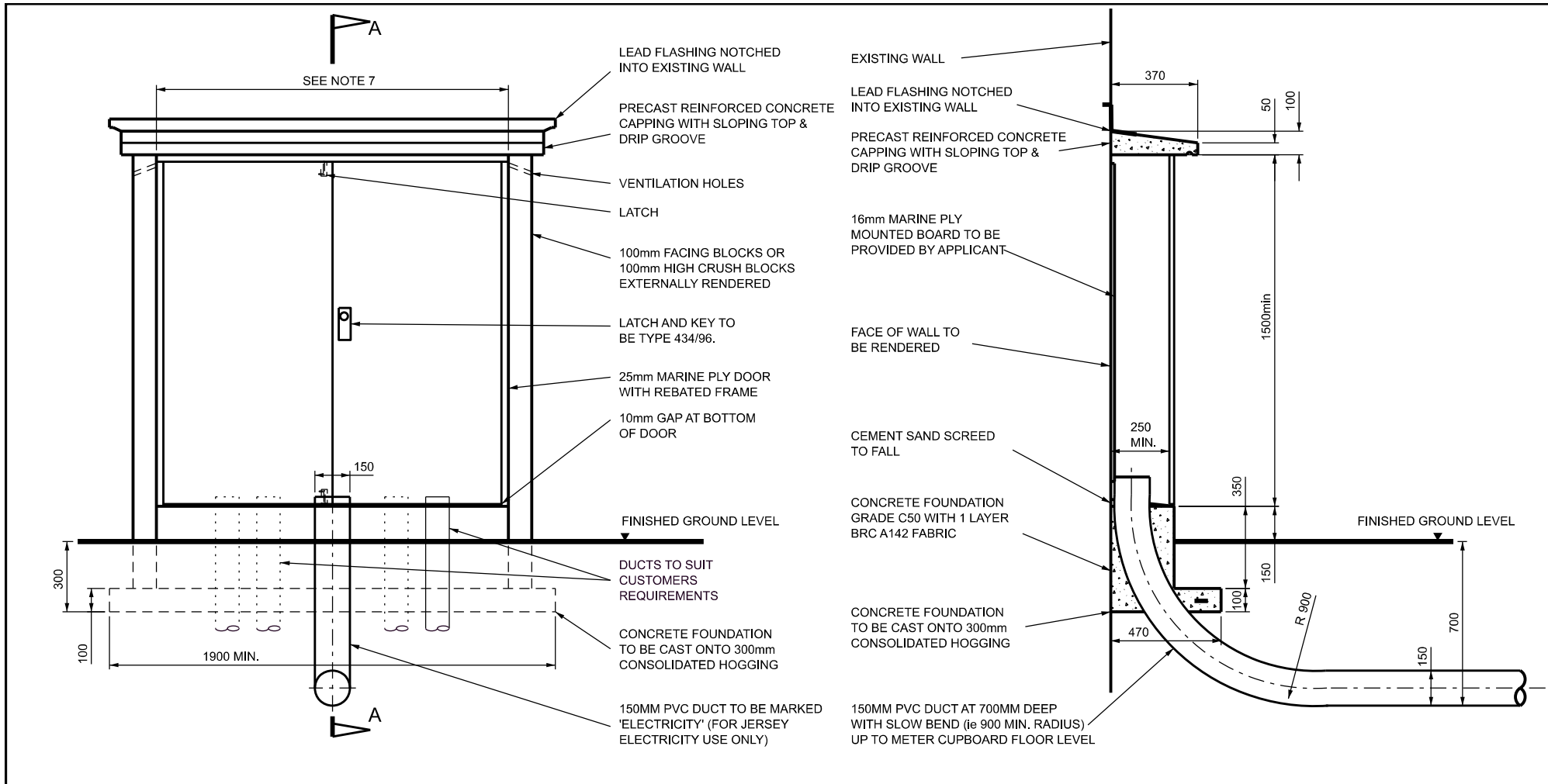
SECTION A-A
